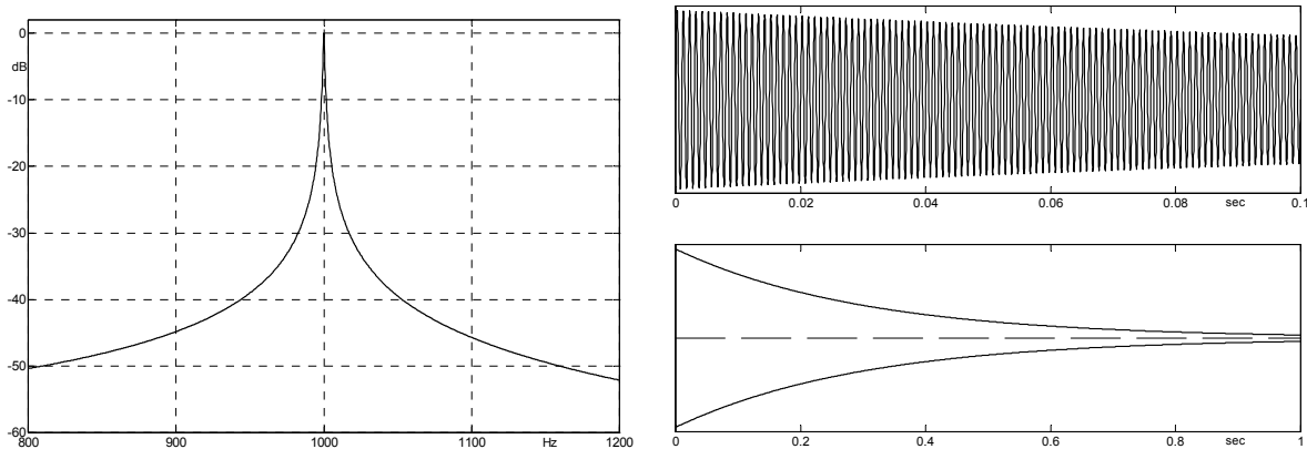
Abb. 0.3: Abklingende Sinusschwingung, f = 1000 Hz, Zeitkonstante \tau = 0,3 s.
