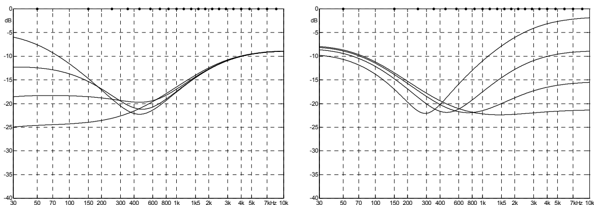
Abb. 0.2: Klangregelung eines Fender-Verstärkers (Übertragungsmaß). Die Punkte am oberen Bildrand markieren das Frequenzgruppenraster (Abszissendiskretisierung zur Schärferechnung).
