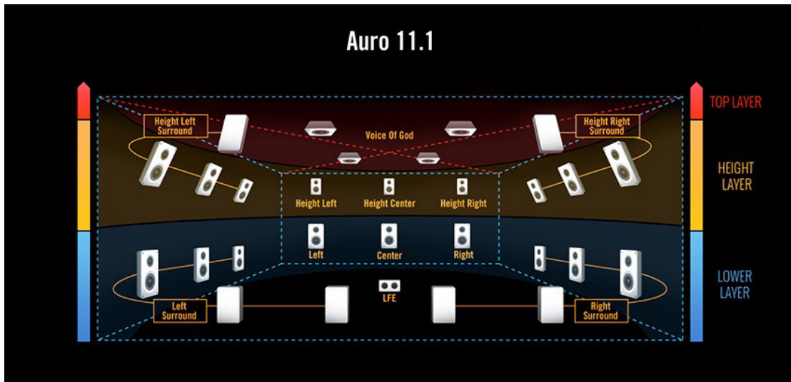
Abbildung 1.22: Auro-3D Anordnung für 11.1 55
