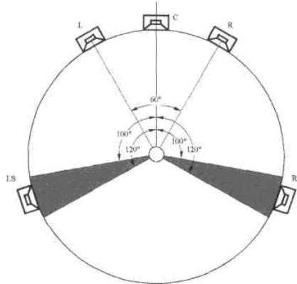
Abbildung 1.18: Referenz-Lautsprecheranordnung mit Winkelangaben nach ITU-775 46
