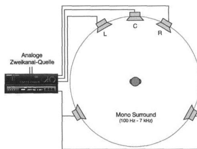
Abbildung 1.17: Wiedergabegerechte Abhörlösung nach ITU-775 44
