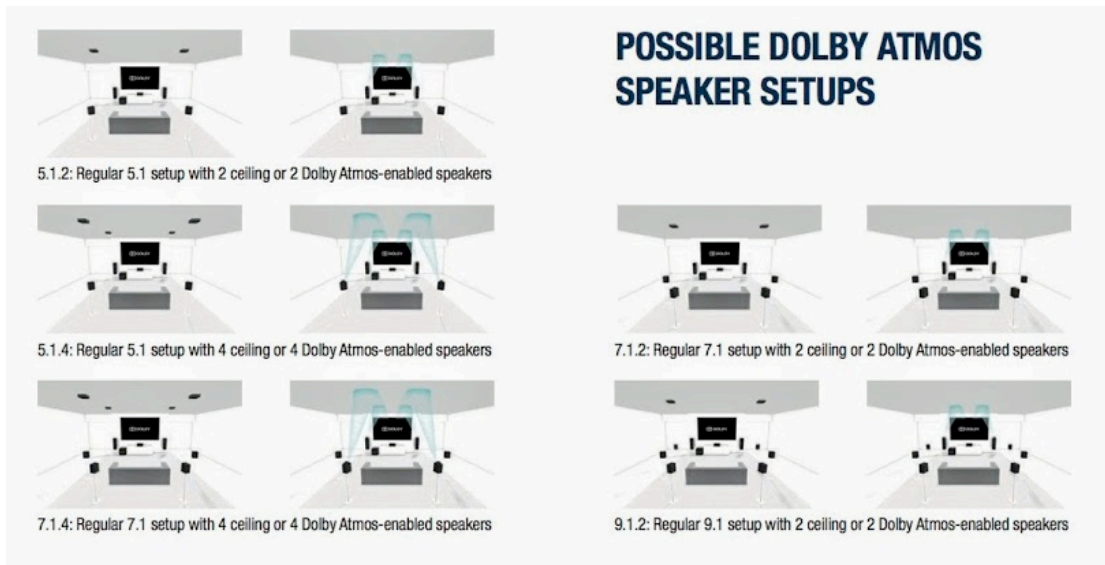
Abbildung 1.23: Dolby Atmos Anordnungen 58
